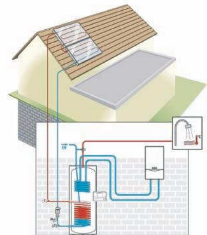
Solarni sistem brez ekspanzijske posode
